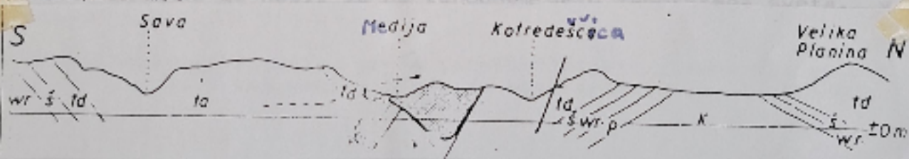
PREREZ SKOZI POSAVSKE GUBE ZAHODNO OD ZAGORJA
